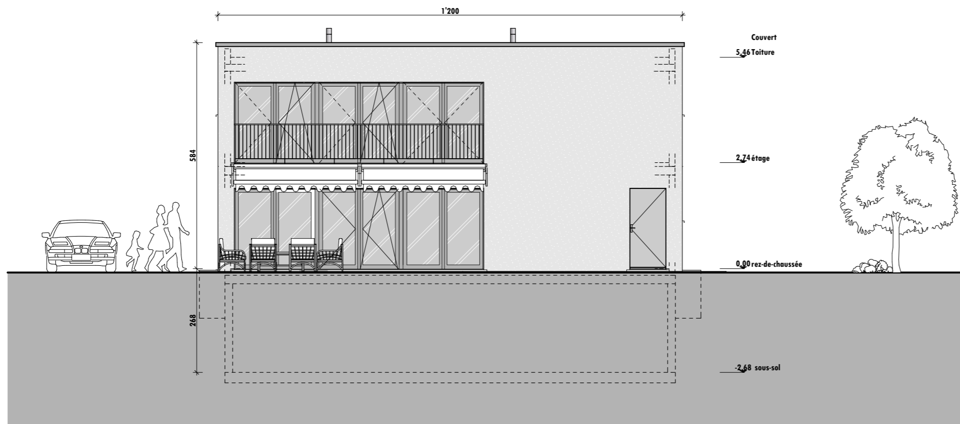
8 façade sud
